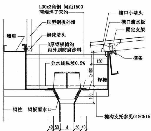
⑫ 咬边连接
