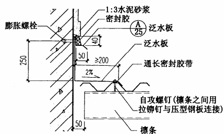
29 紧固件连接
