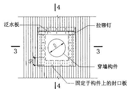
构件穿墙做法二 (用于 D \geq 1000 )
