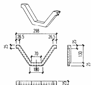
W600型屋面檐口装饰板
