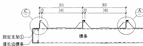
YX51-360 (角弛Ⅱ) 型压型钢板横向连接
