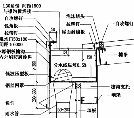
⑦ 紧固件连接
