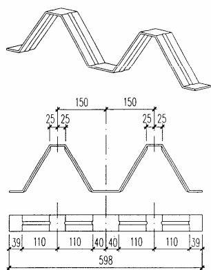
W600型屋面板固定支架(中间)
