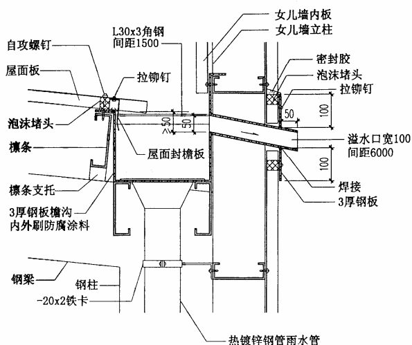
⑩ 紧固件连接
