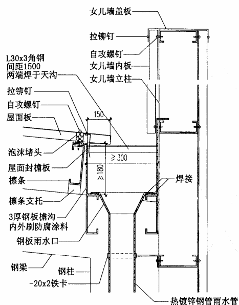
⑨ 紧固件连接
