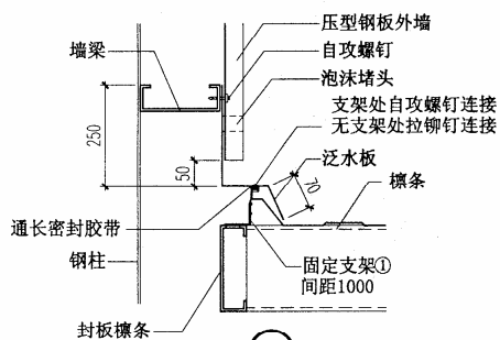
27 咬边连接
