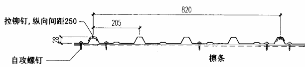
YX28-205-820 型墙面压型钢板横向连接
