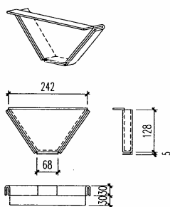
W600型屋面泛水堵头板
