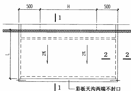
雨棚平面图
