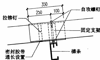
W600 型彩色钢板屋面纵向搭接
