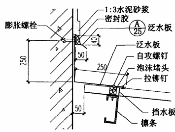
30 紧固件连接
