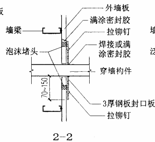
构件穿墙做法二 (用于 D \geq 1000 )
