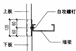
墙面压型钢板纵向搭接
