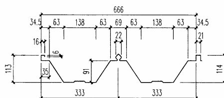
YX114-333-666 型压型钢板
