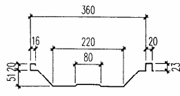
YX51-360 (角弛 II) 型压型钢板
