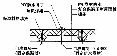
屋面横向搭接示意
