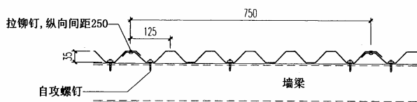
YX35-125-750 (V125) 型墙面压型钢板横向连接
