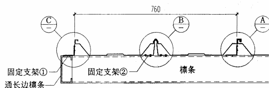
YX51-380-760 (角弛Ⅲ) 型压型钢板横向连接
