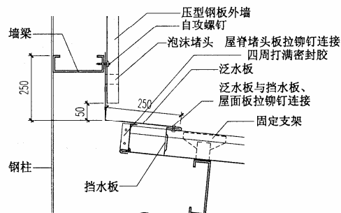
28 咬边连接
