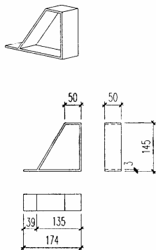
W600型屋面板固定支架(端部)
