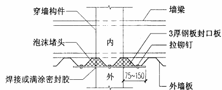
构件穿墙做法一
