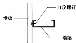
墙面压型钢板纵向连接
