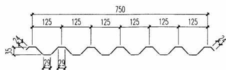
YX35-125-750 (V125) 型压型钢板
