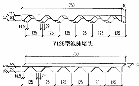
V125型挡水板 (S为板厚)
