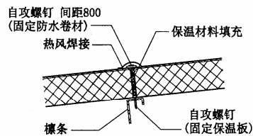
屋面纵向连接示意
