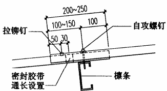
V125 型彩色钢板屋面纵向搭接
