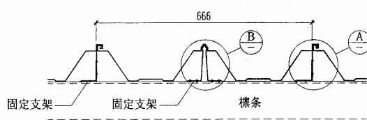
YX114-333-666 型压型钢板横向连接
