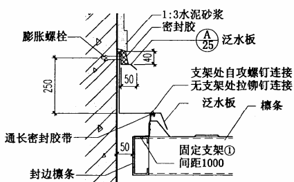
31 咬边连接
