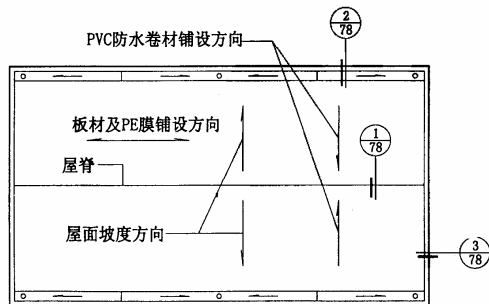
卷材铺设平面示意图
