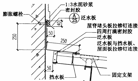
32 咬边连接
