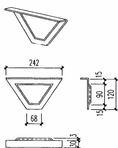
W600型屋面泛水挡水板
