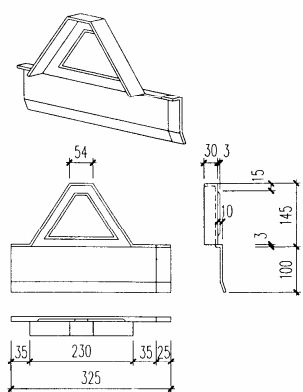
W600型屋面檐口堵头板(中间)
