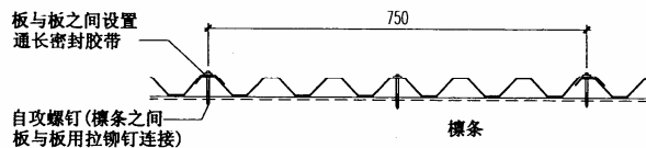
YX35-125-750 (V125) 型压型钢板屋面横向连接一 (宜用于屋面防水要求较低、单坡长度较小及半开敞式建筑物)
