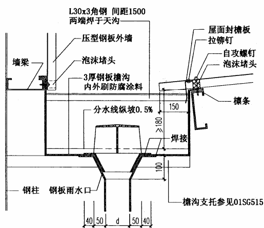
⑪ 紧固件连接
