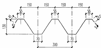
YX130-300-600 (W600) 型压型钢板
