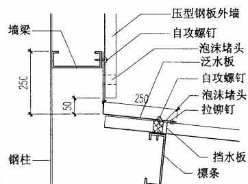
26 紧固件连接
