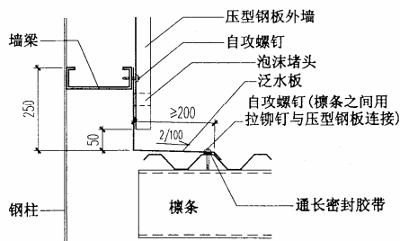
25 紧固件连接
