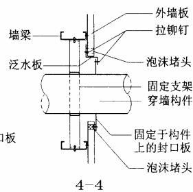
构件穿墙做法二 (用于 D \geq 1000 )
