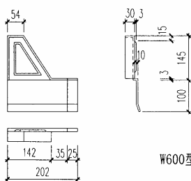
W600型屋面板固定支架(中间)
