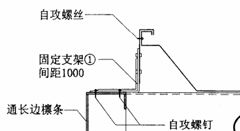
压型钢板屋面隐藏式咬边连接详图
